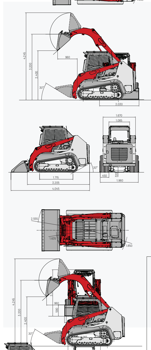
TL12R-2 dimenzije (mm)
