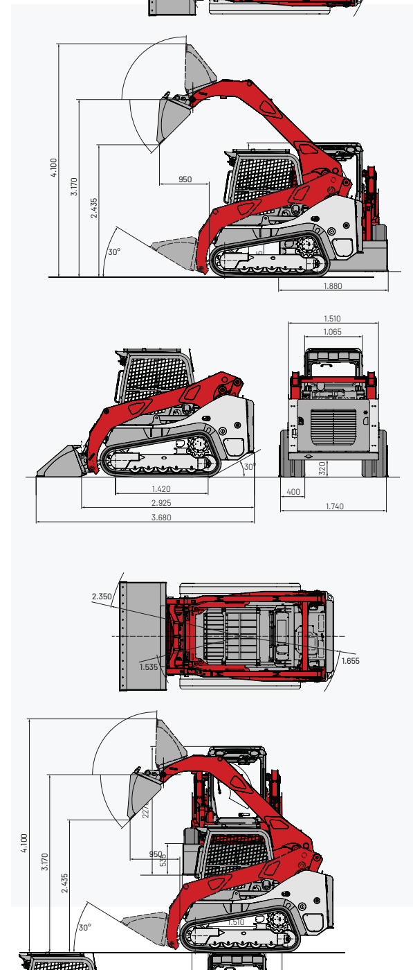
TL10V-2 dimenzije (mm)
