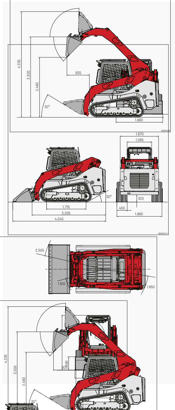
TL12V-2 dimenzije (mm)
